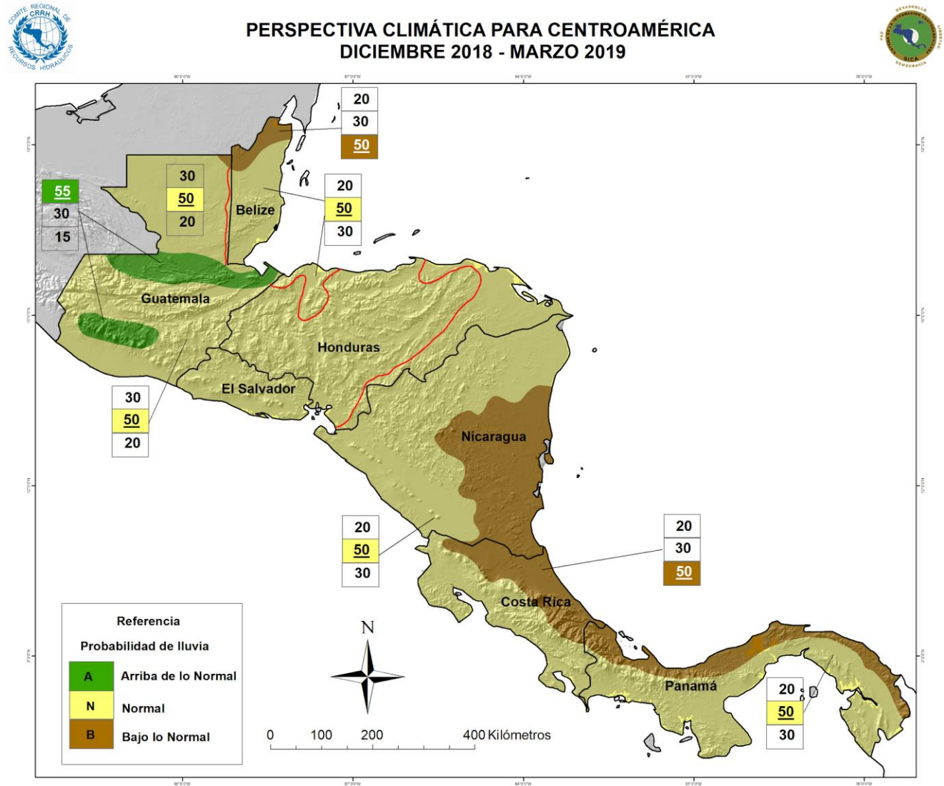
Figura 1. Mapa de la Perspectiva del Clima para Centroamérica, diciembre 2018, enero,
